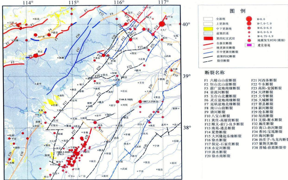
图2-2 区域地震构造体系图
